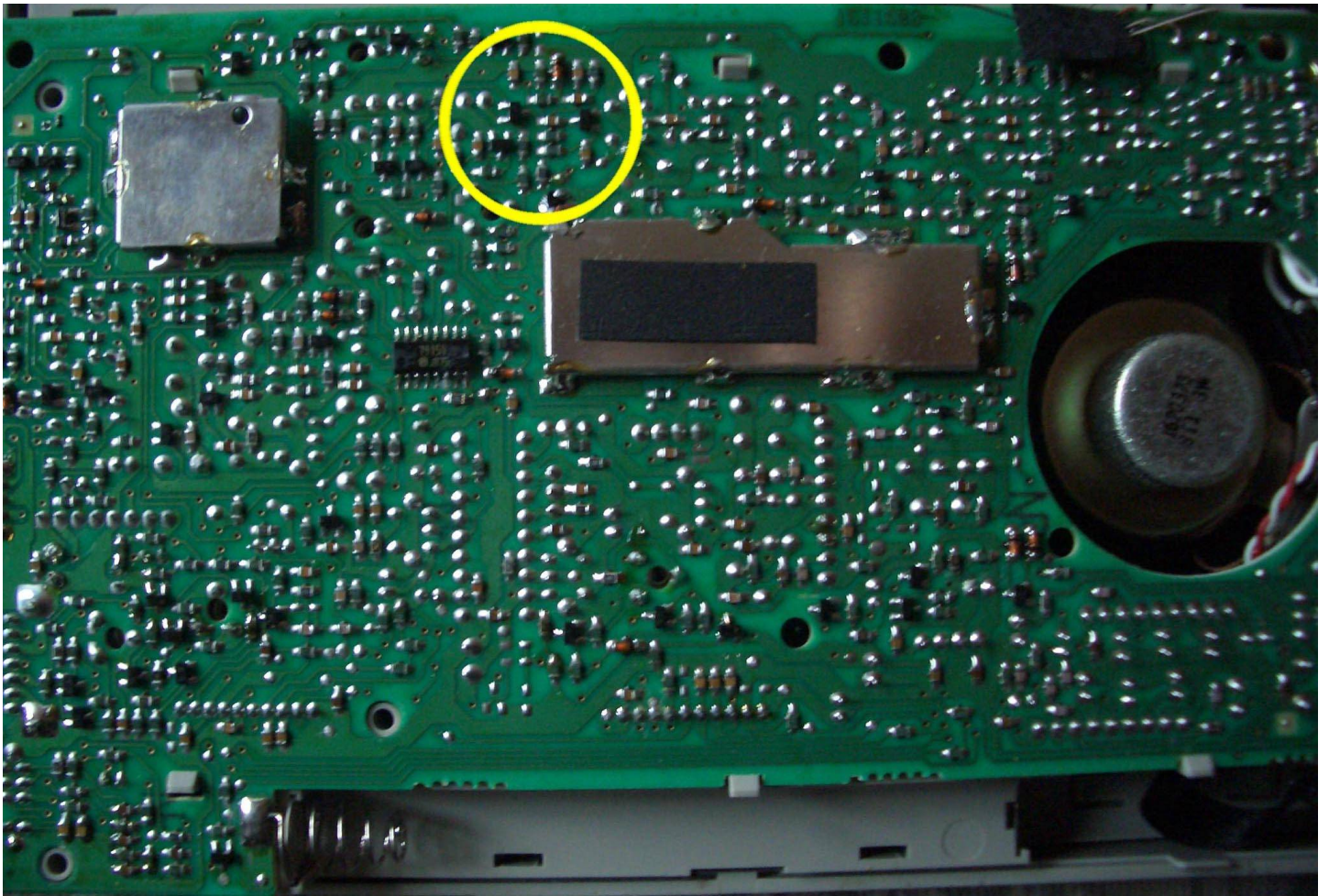
Bild 3: Hauptplatine (Lage des ZF-Abgriffspunktes)
