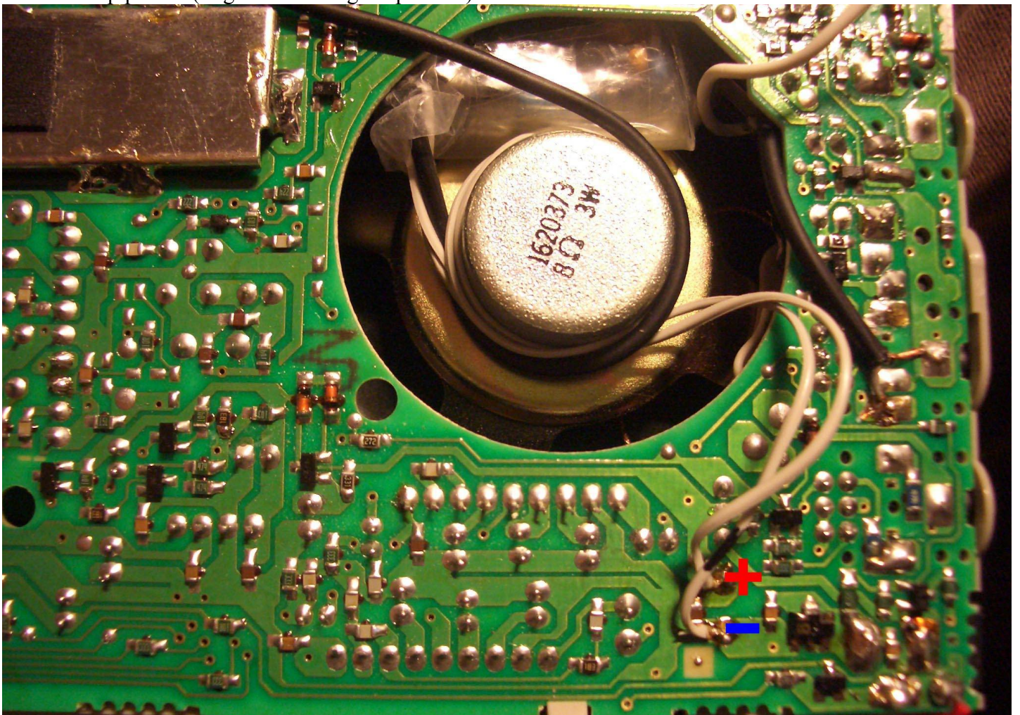
Bild 4: Hauptplatine (Versorgungsspannung und Mischerplatine am Lautsprecher)
